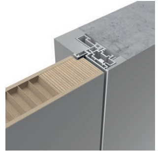
INVISIBLE frame
