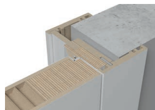
UNIDOOR frame
